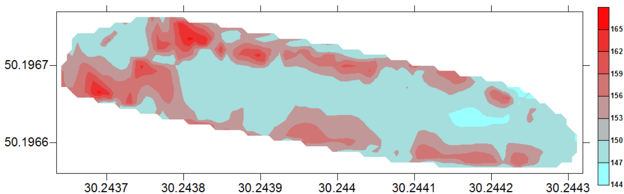
Рис. 8 – Картограма питомого опору ґрунту за результатами вимірювань голчастим способом.
