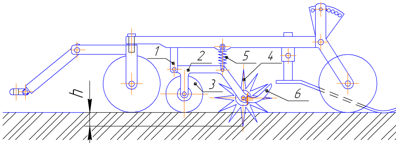
Рис. 5 – Польова установка із голчастими дисками
