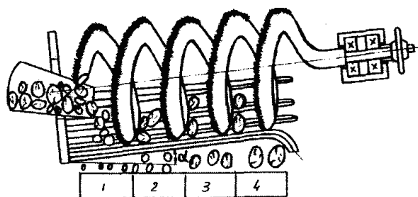
Решітчасто-гвинтова сортувалка
