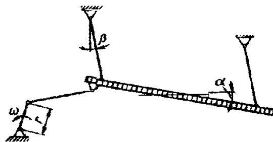
Грохотна сортувальна поверхня
