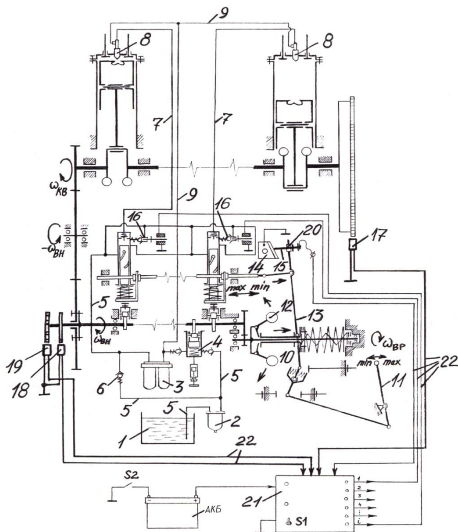
Рис. 1 Схема системи автоматичного регулювання потужності багаточиліндрового двигуна
