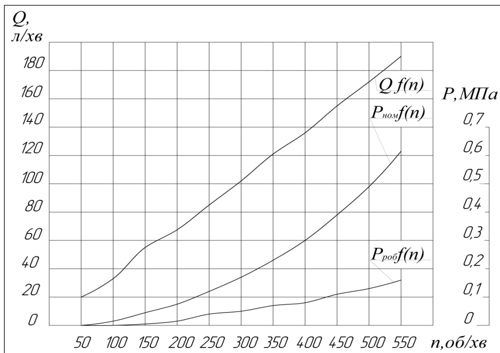
Рис. 3. Гідравлічна характеристика відцентрового насоса АН – 5
