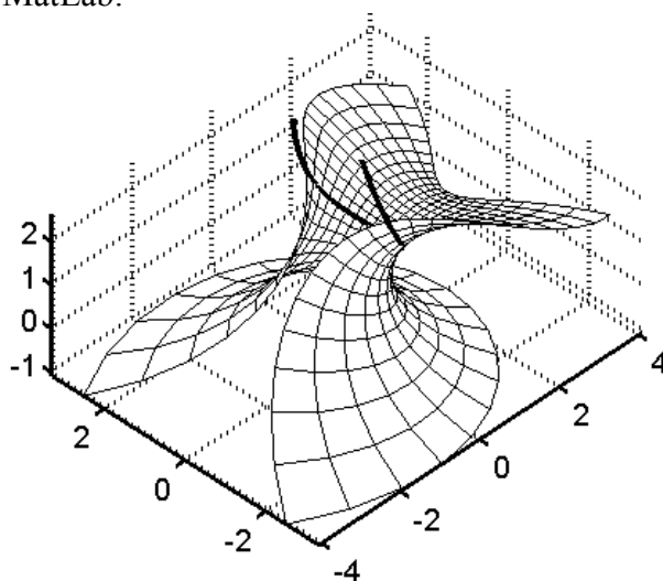
Рис. 8. Приклад побудови мінімальної поверхні.
