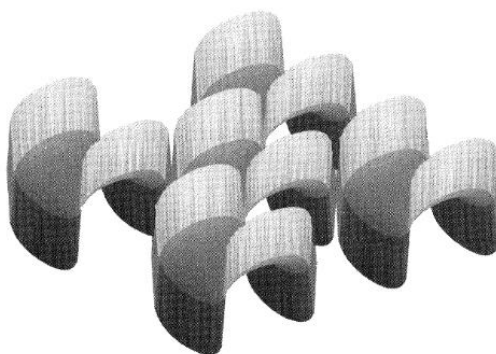
Рис.4. Поверхня Шерка.
